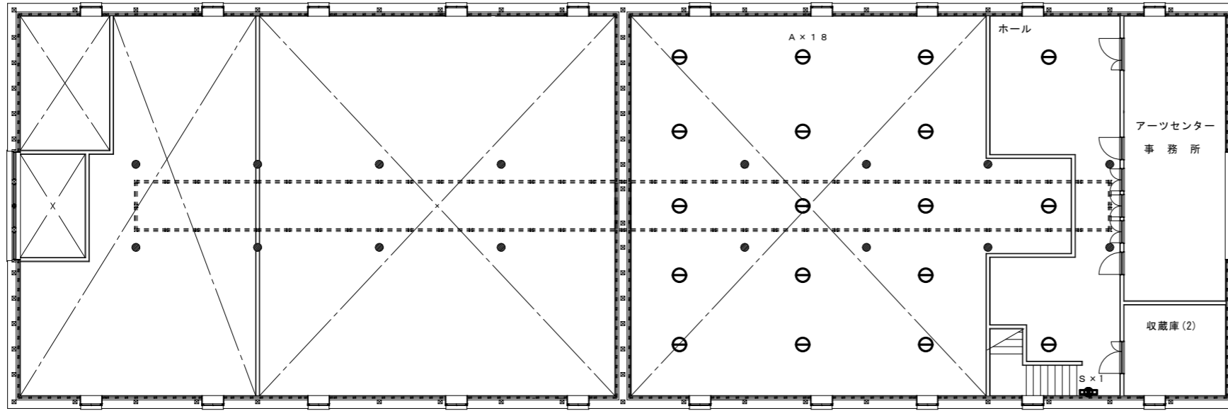
2階平面図 (1:100)
